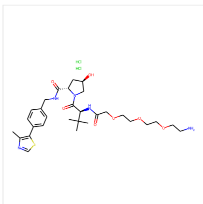
Structure VH 032 amide-PEG3-amine, CAS 2376990-24-6
