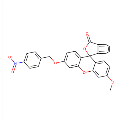
Structure CAY10730, CAS 2206677-06-5
