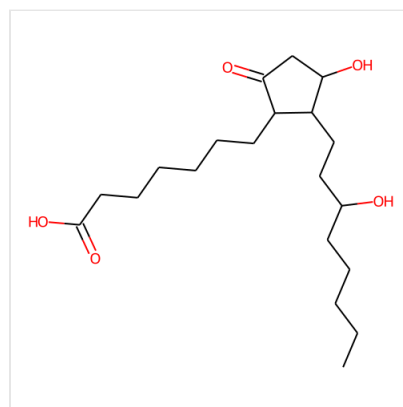
Structure 13,14-dihydro Prostaglandin E1, CAS 19313-28-1
