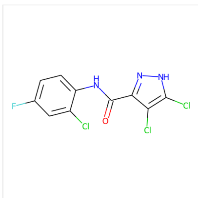
Structure BLX3887, CAS 934758-70-0
