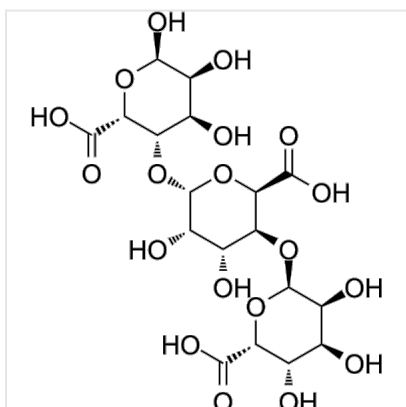
Structure L-Triguluronic acid, CAS 66754-14-1
