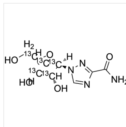
Structure Ribavirin-13C5, CAS 1646818-35-0
