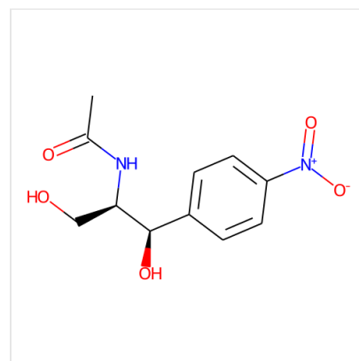
Structure Corynecin I, CAS 4423-58-9
