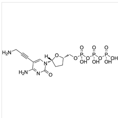
Structure 5-Propargylamino-ddCTP, CAS 114748-56-0
