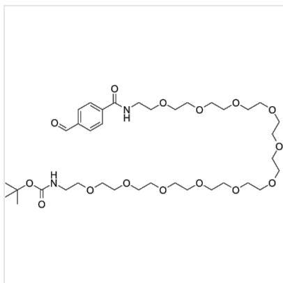
Structure Ald-Ph-amido-PEG11-NH-Boc, CAS 1245813-70-0
