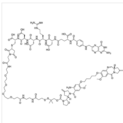
Structure EC2629, CAS 2245361-43-5
