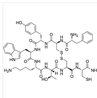
Structure Nendratareotide, CAS 2251119-65-8
