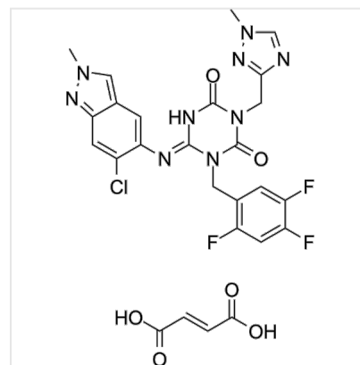
Structure Ensirelvir fumarate, CAS 2757470-18-9
