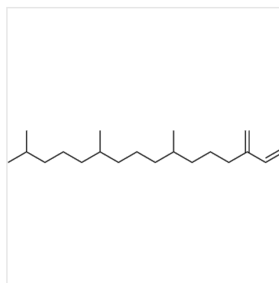
Structure Neophytadiene, CAS 504-96-1
