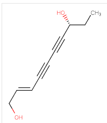
Structure R,E)-Deca-2-ene-4,6-diyne-1,8-diol, CAS 931116-24-4
